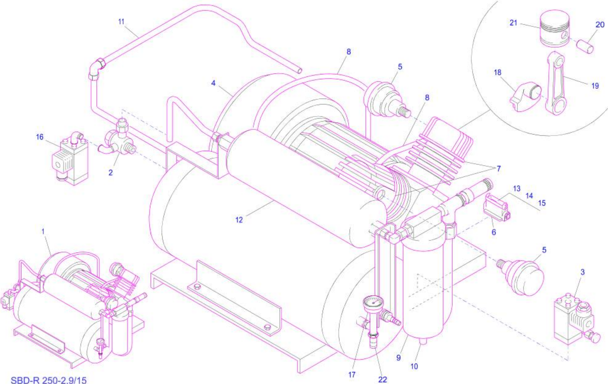
SBD-R 250-2,9/15
