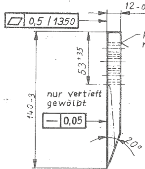
Ansicht Y M 1:2,5
