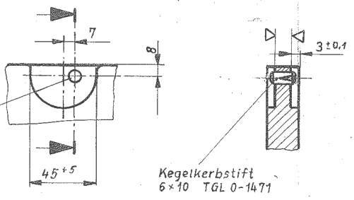
Einzelheit Z M 1:2,5
