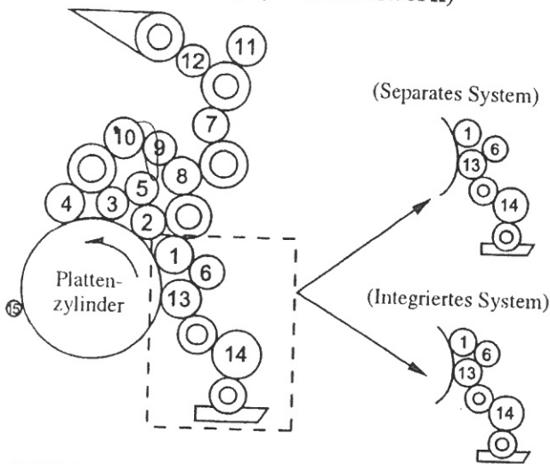
(1., 3. Druckwerk)
