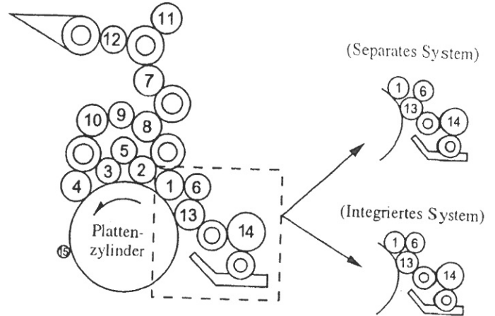
(2., 4. Druckwerk)
