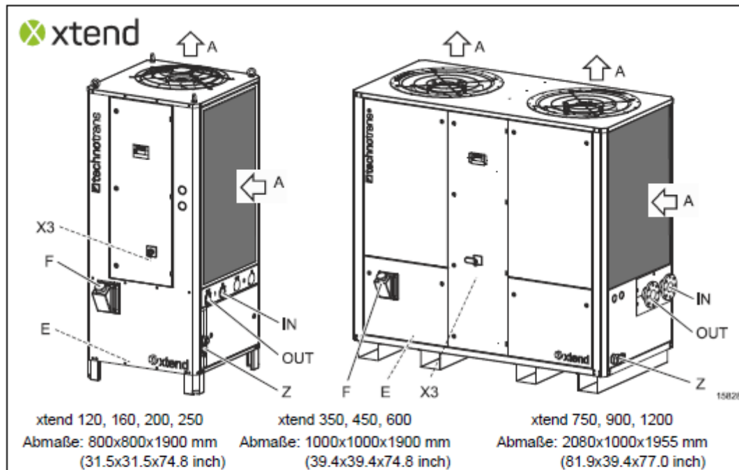
Abb. 1: Luftgekühlte Version (A) (Beispiel)
